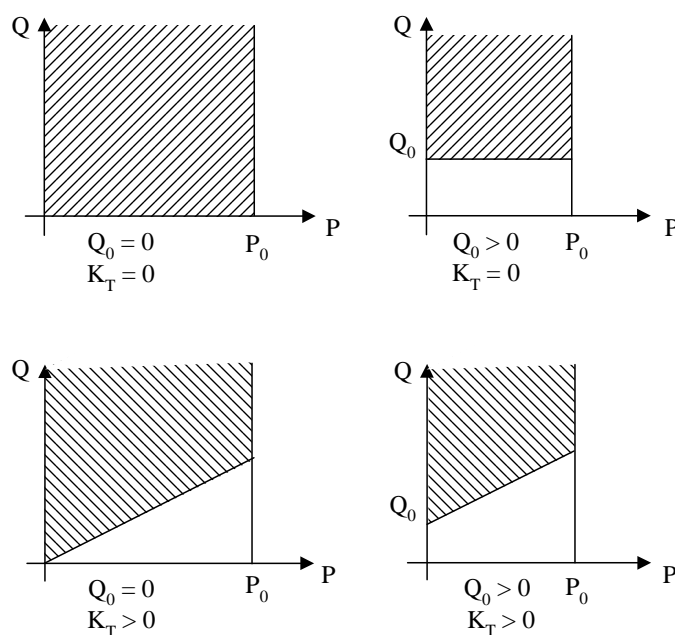
Рисунок 1.3.1 - Зоны срабатывания по реактивной мощности
