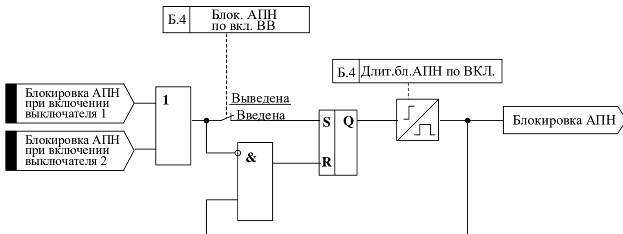
Рисунок 1.3.3 – Функциональная схема формирования внутреннего логического сигнала "Блокировка АПН"
