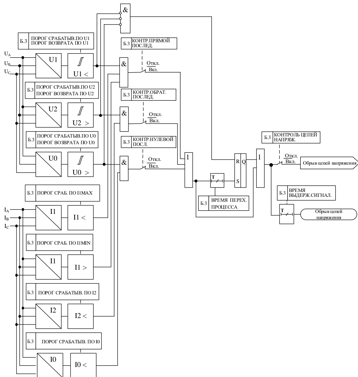
Рисунок 1.3.5 – Функциональная схема контроля цепей напряжения
