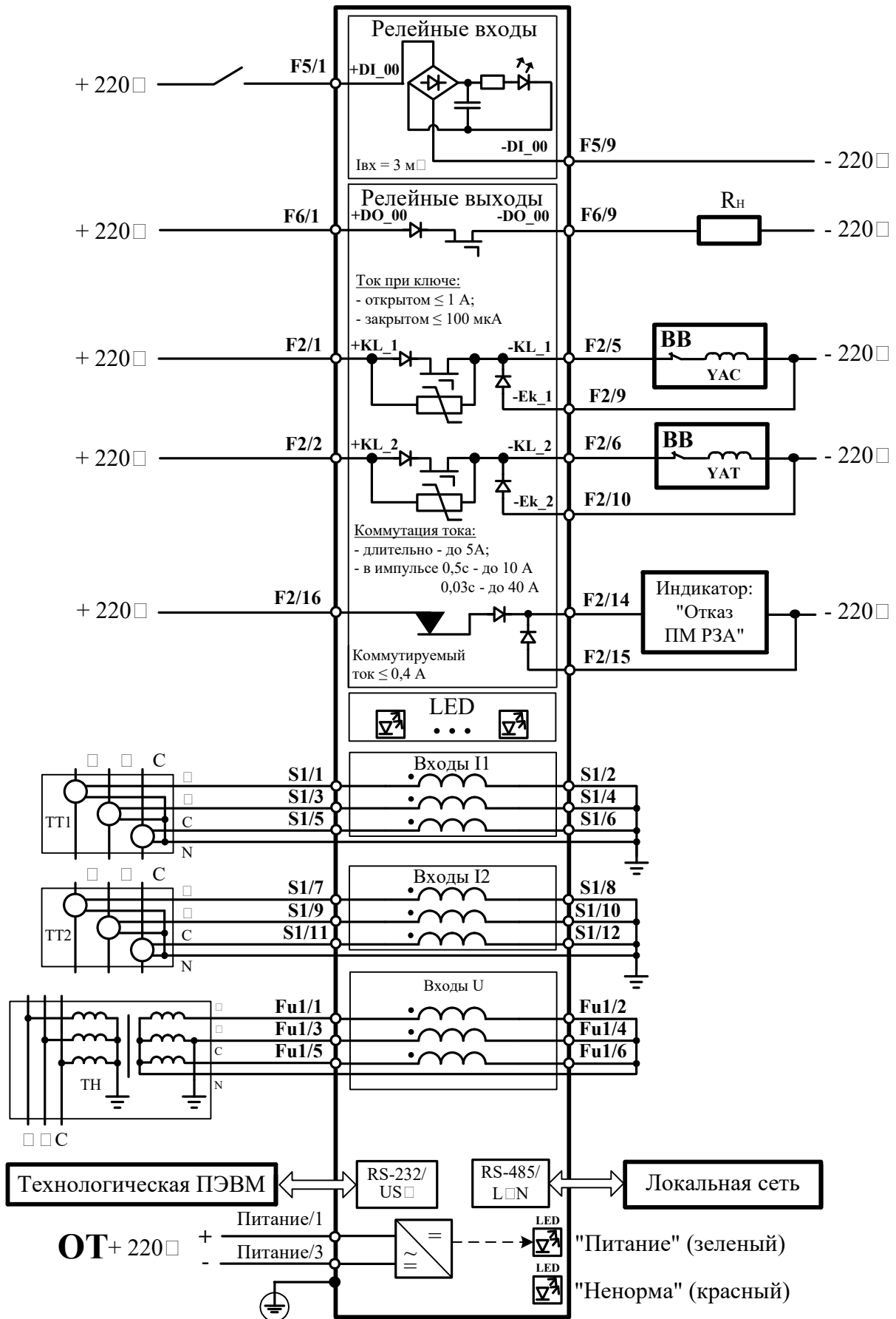
Рисунок 1.2.2 - Типовая схема внешних подключений ПИМ РЗА
