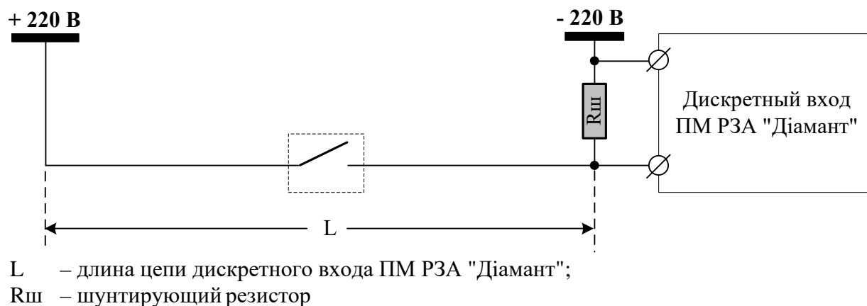
Рисунок 1.2.1 – Пример установки шунтирующего резистора
