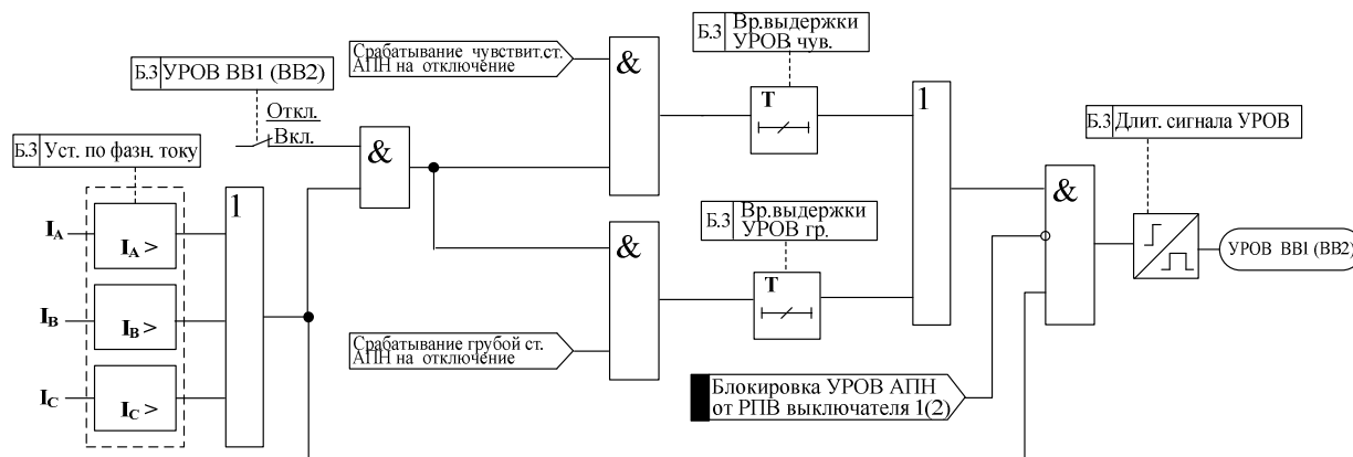
Рисунок 1.3.4 - Функциональная схема УРОВ ВВ1 (ВВ2)
