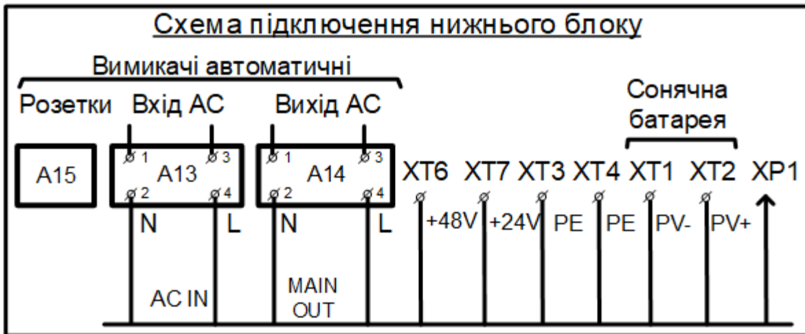
Рисунок 7 – Схема підключення нижнього блоку.
